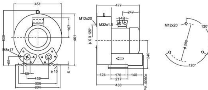
Lajac blower installation parameter
