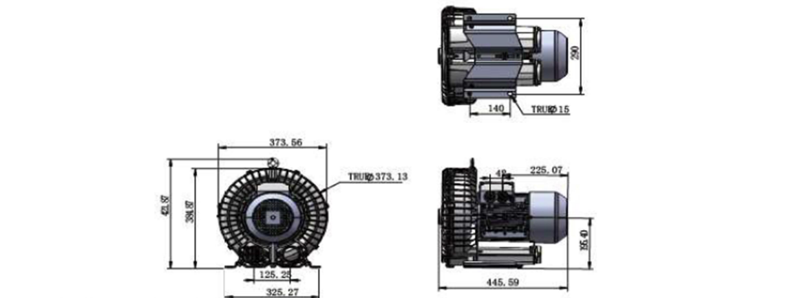
Lajac blower installation parameter
