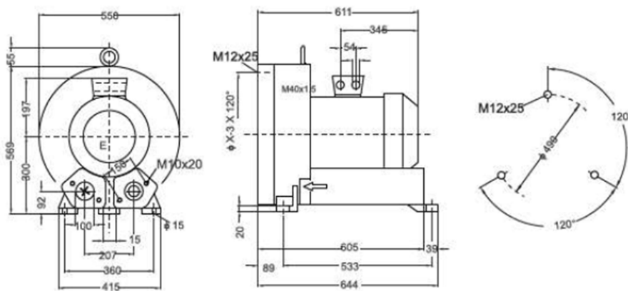
Lajac blower installation parameter
